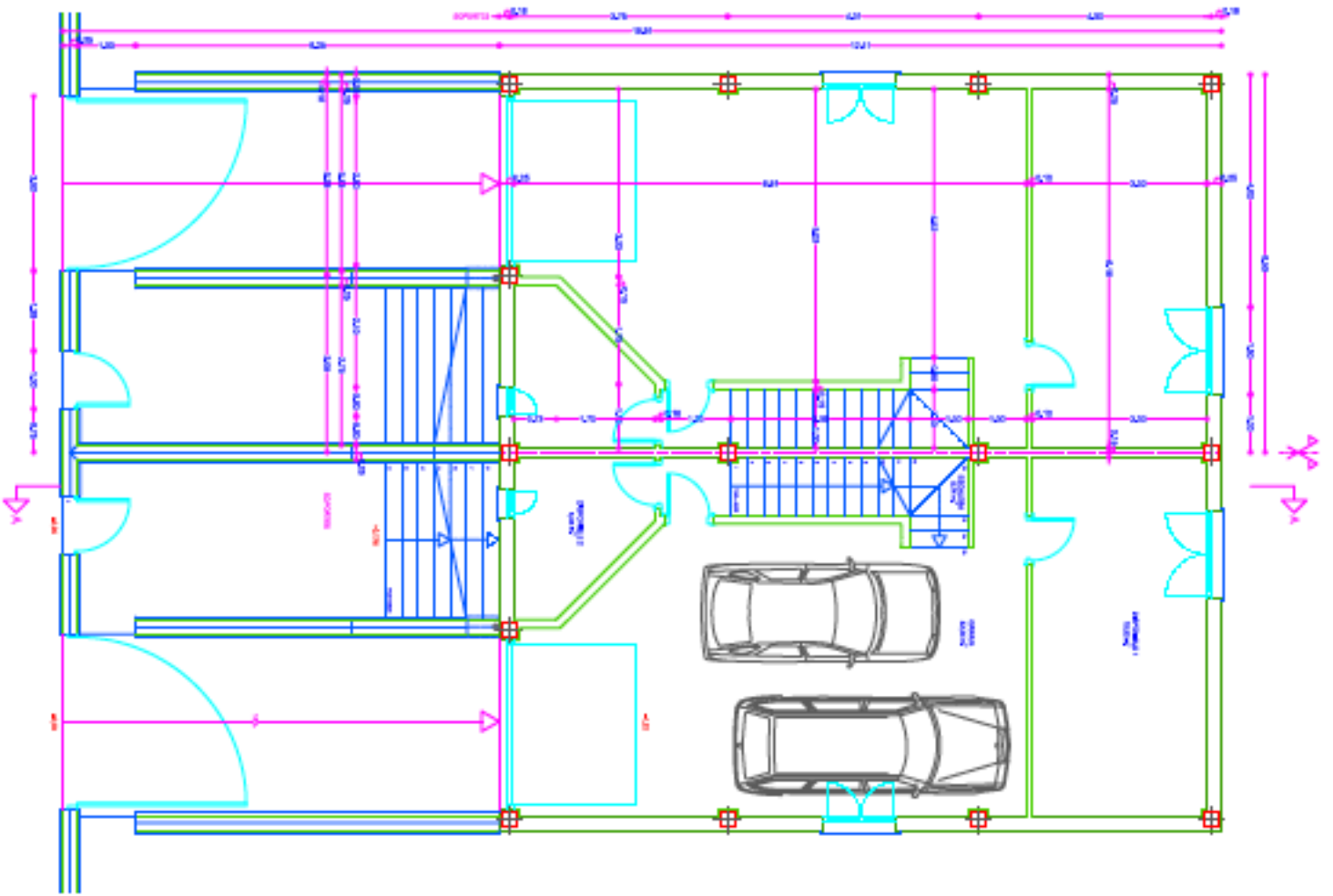
PLANTA SEMISOTANO
