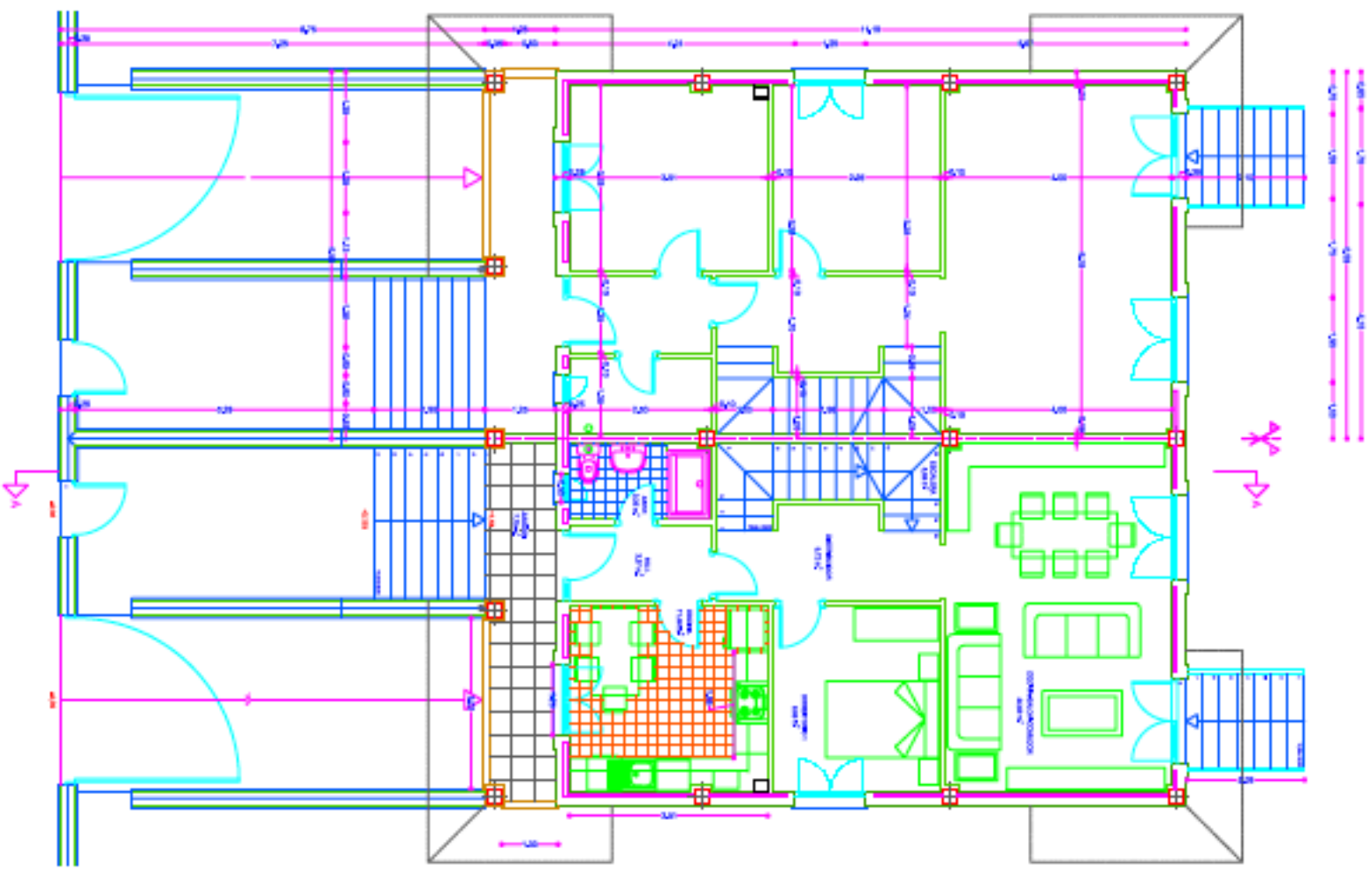
PLANTA BAIA
